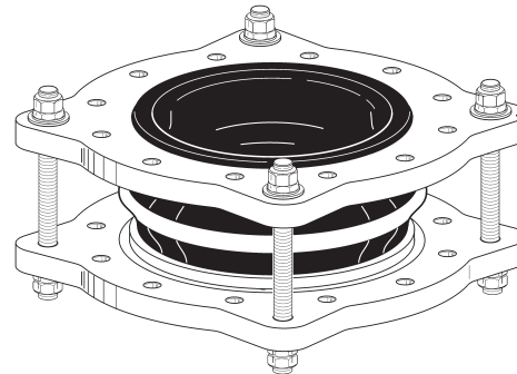
Tirants avec limitation extérieure avec coupelle sphérique et bague conique Type ... ZS (jusqu'au/from DN 350) Tie rods with outer limitation in spherical discs and conical seats
