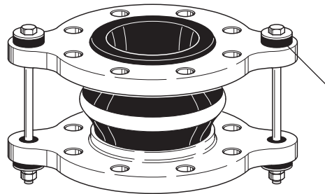
Tirants avec limitation extérieure et amortisseurs en caoutchouc Type ... ZS (jusqu'au/up to DN 300) Tie rods with outer limitation in rubber bushings
