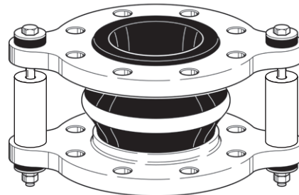
Tirants avec limitation intérieure et extérieure Type ... ZSS (bis/up to DN 300) Tie rods with inner and outer limitation
